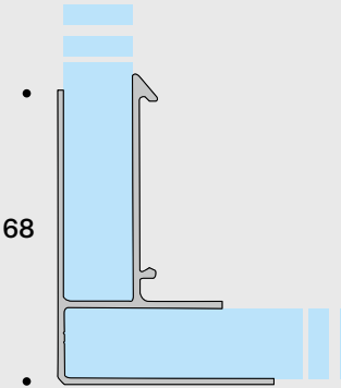
Profilo F2 Angolare Profile F2 Angular Profil F2 Angulaire
