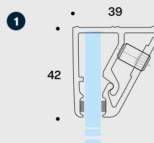
Profilo a muro Wall profile Profil de mur
