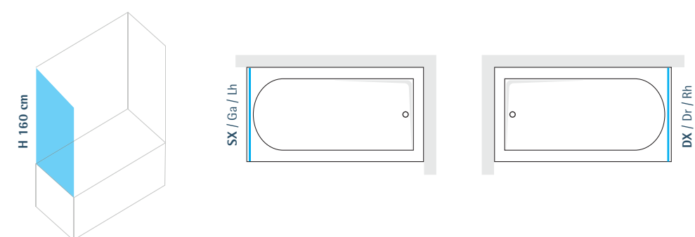
LATO FISSO CON PROFILO ANGOLARE / Paroi fixe avec profilé angulaire / Fixed glass with angular profile H 160 cm
