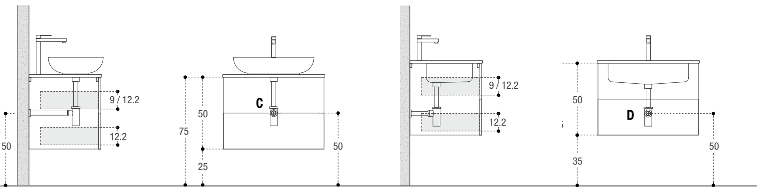
Posizionamento scarichi con cassetto scansato Drain position on washbasin base units with drawer undertop Position écoulement sur éléments bas lavabo avec tiroir sous lavabo
