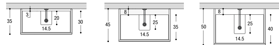
Posizionamento scarichi con cassetto scansato Drain position on washbasin base units with drawer undertop Position écoulement sur éléments bas lavabo avec tiroir sous lavabo
